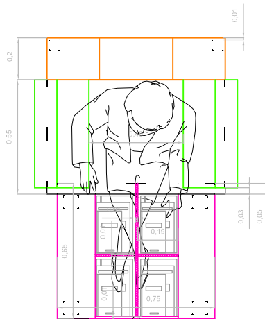
Planta (Desplaçat)
