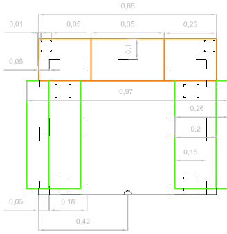
Planta (Recollit)
