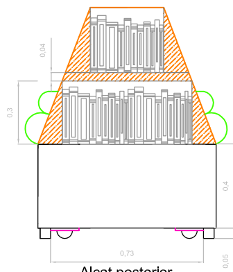
Alçat posterior
