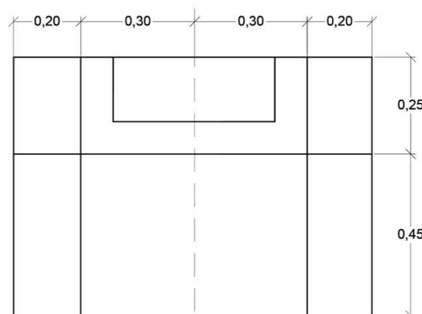
PLANTA SUPERIOR
